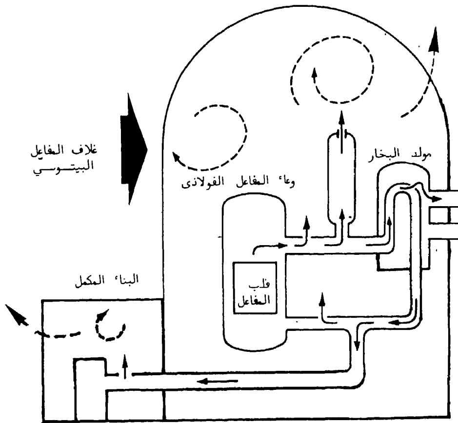
الشكل (٤) بيان مبسط لاحتمال حدوث خطر في مفاعل الماء الخفيف المضغوط وسنارب نواتج الوقود المشطرة
